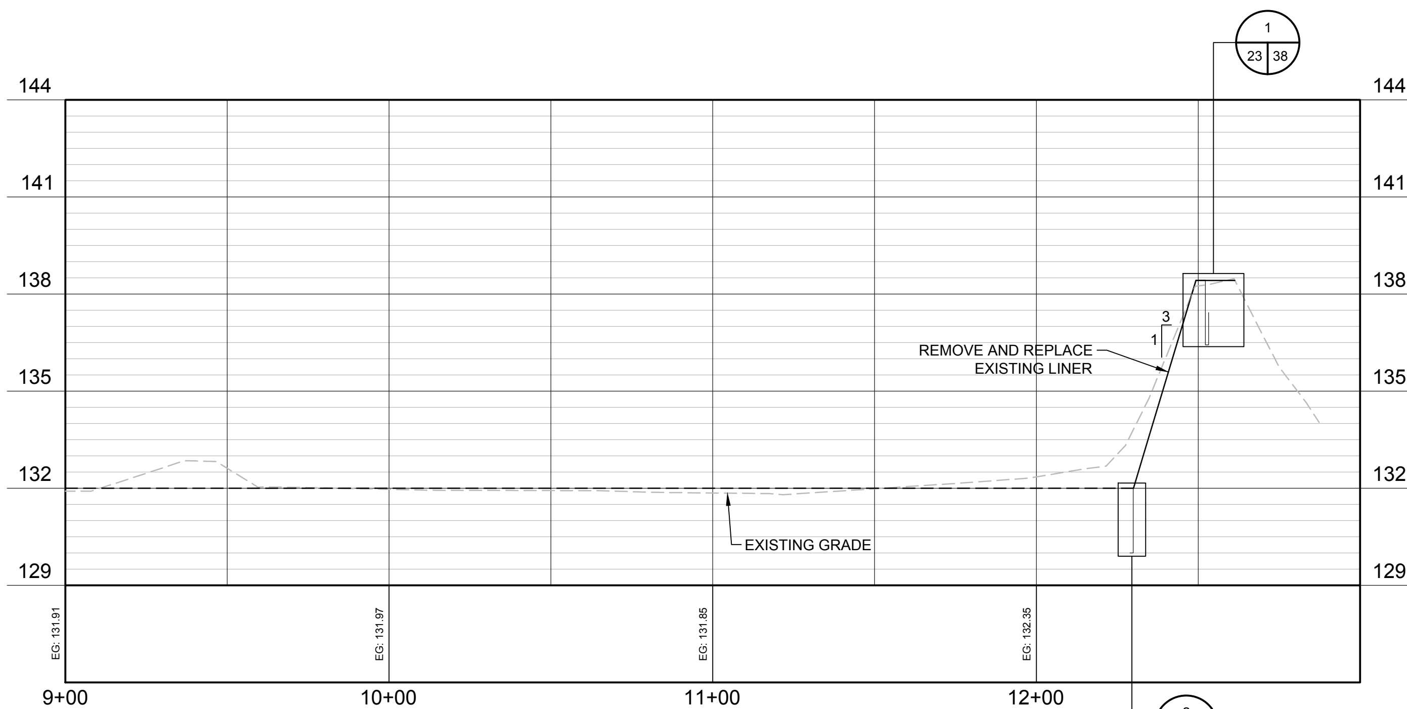
RIB 5 SECTION SCALE: 1" = 30' H 1" = 3' V
