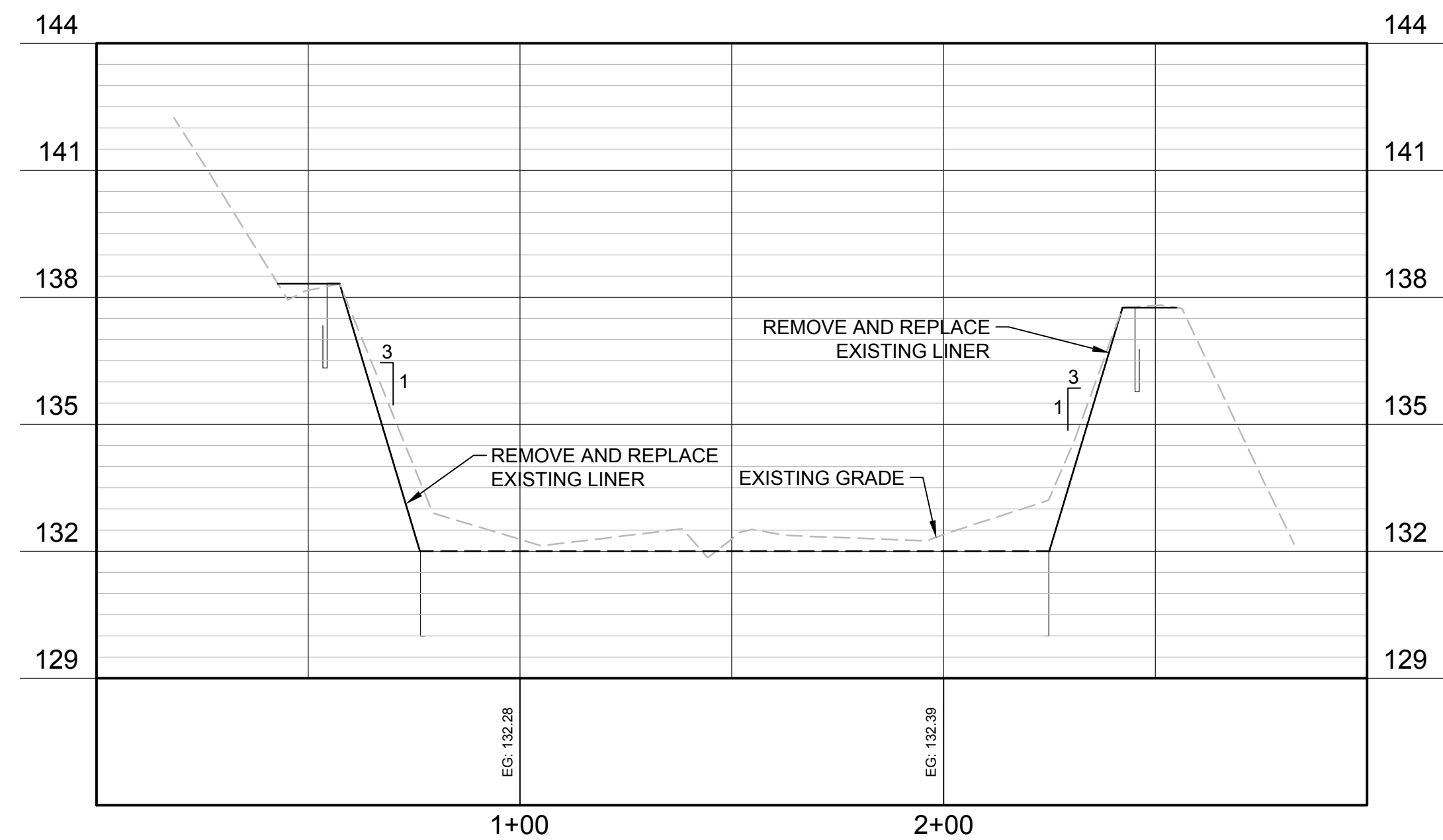
RIB 5 SECTION SCALE: 1" = 30' H 1" = 3' V
